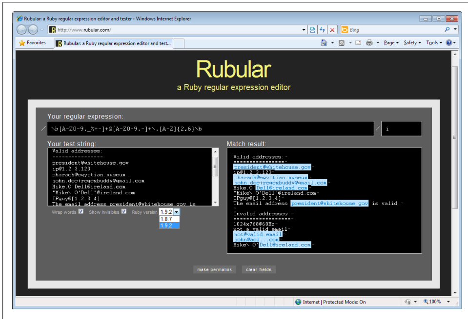
Figure 1-5. regex.larsolavtorvik.com
