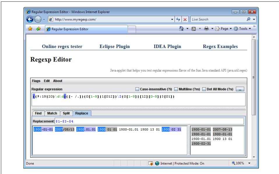
Figure 1-8. myregexp.com
